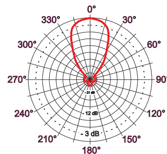
UMTS (1920-2170 MHz)
